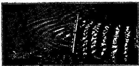
ציור 7 עקיפה: הזית-גלים ישרה (הבאה מימין) נעכבת ע"י מחיצה; הנקב שממש מרכזו לסערכת-גלים מעגלית (המתפשטת שמאלה)
